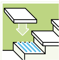
Lepení schodnic na betono- vý podklad
